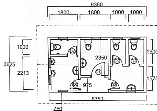
TOILET UNIT PLAN
